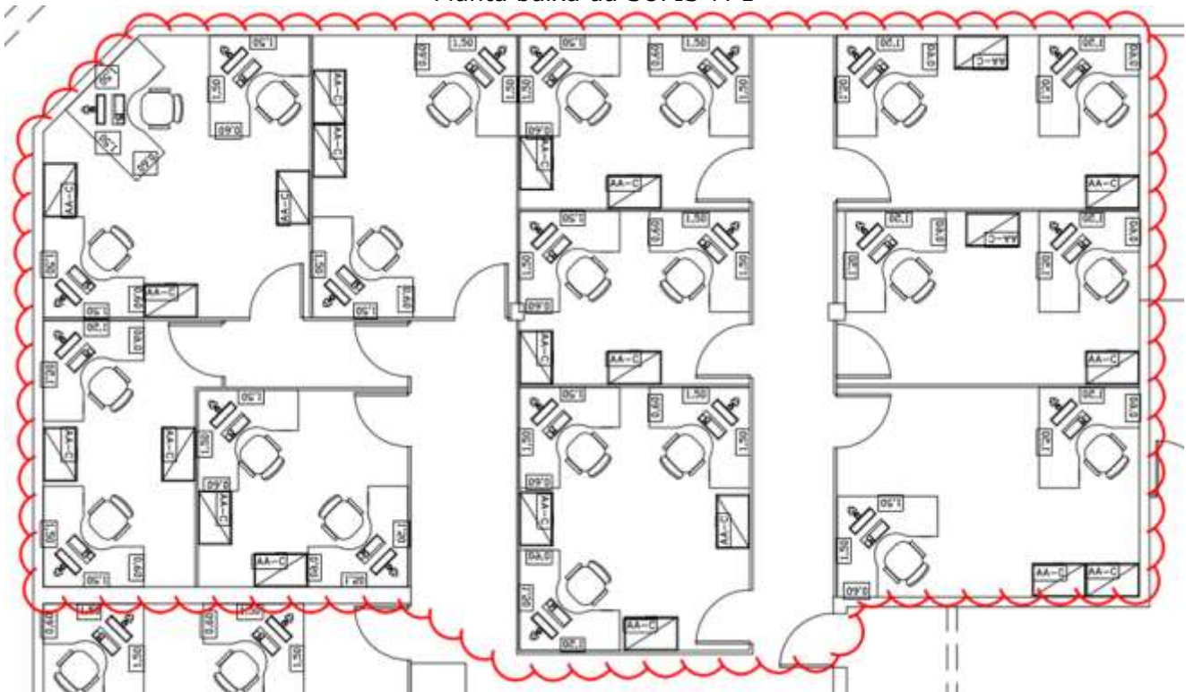
Planta baixa da SUFIS-M 1
